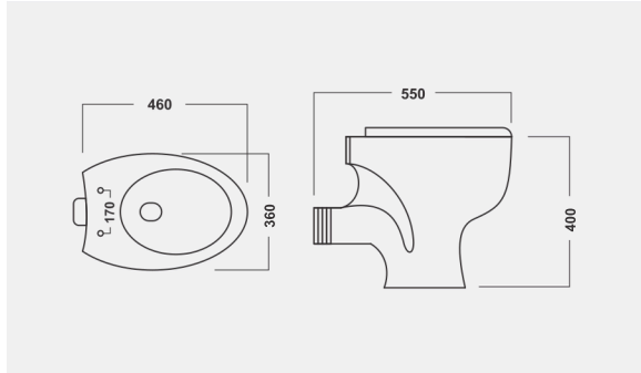
▶ RUBIA E.W.C. 460x360x400mm P-Trap
