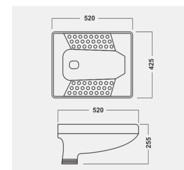
► ORISSA PAN 20" (AQUA)
