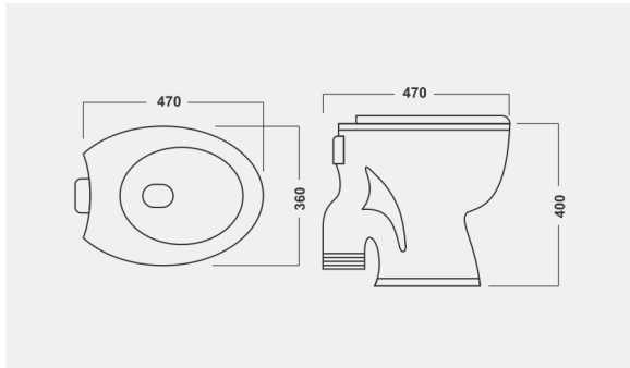
▶ RUBIA E.W.C. 470x360x400mm S-Trap
